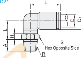
90° Elbow XZC21
